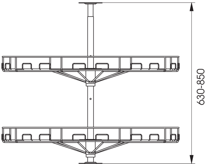
Koottu yksikkö
